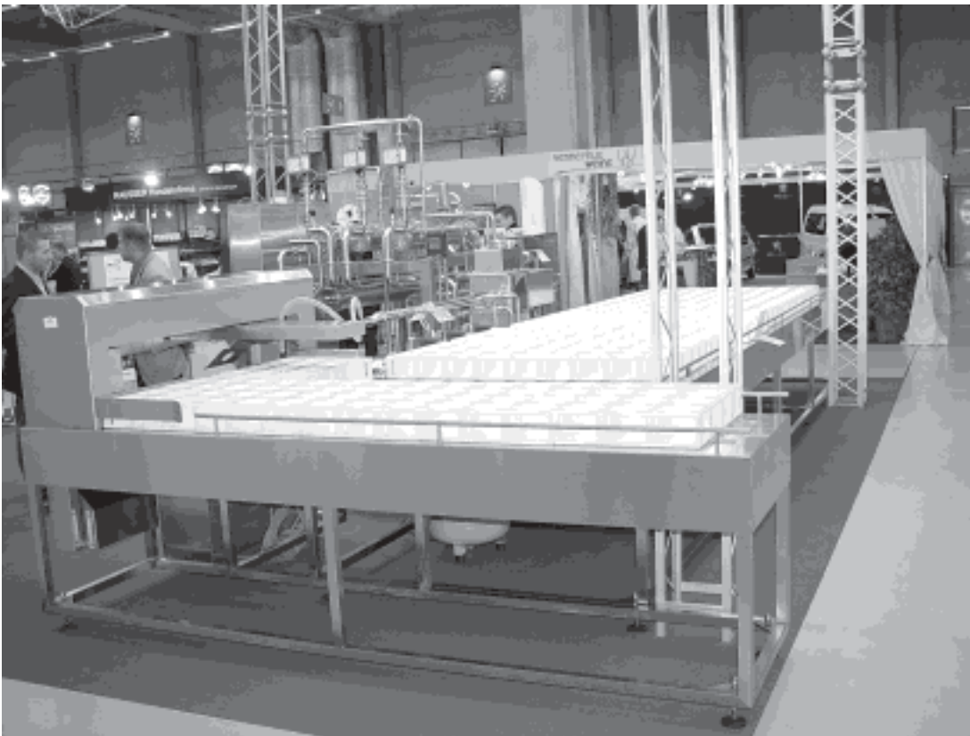
Abb. 5. Die erste anlagentechnische Umsetzung: Prototyp «Cheesemaker 02».
