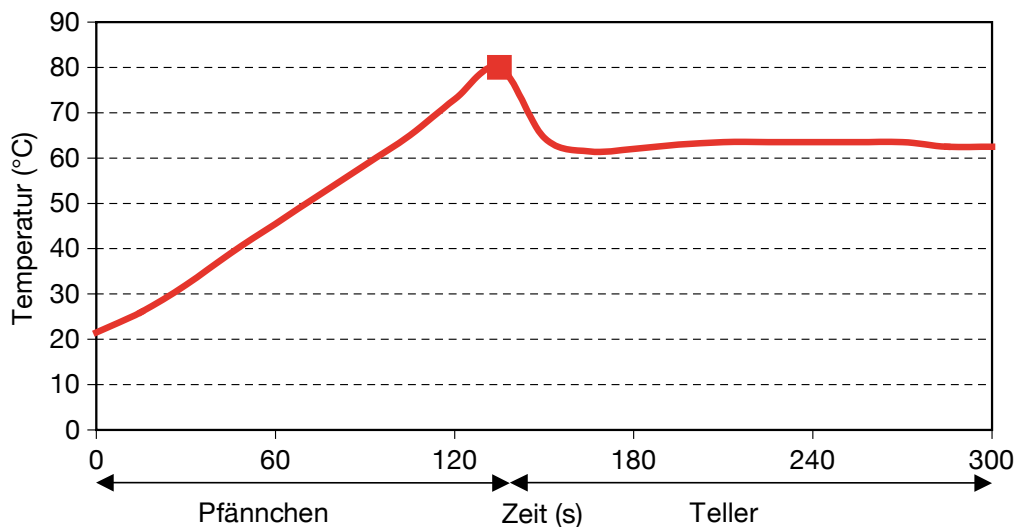
Abb. 1. Temperaturverlauf von Raclette während des Erwärms im Pfännchen und des Abkühlens auf dem Keramiksteller (Mittelwert von 2 Messungen).
