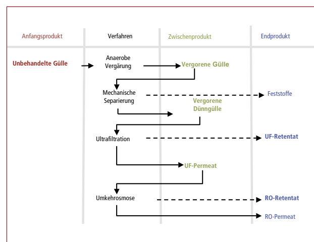
Abb. 1 | Verfahrensschritte der GÜlleaufbereitung zur Erzeugung der verschiedenen Düngerprodukte. Nur die fett geschriebenen Düngerprodukte wurden in den Gefäss- und Feldversuche untersucht.
