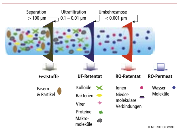
Abb. 2 | Stoffabtrennung mittels Separierung und Membrantrennung (Ultrafiltration, UF und Umkehrosiose, RO) bei der Aufbereitung von Gülle.
