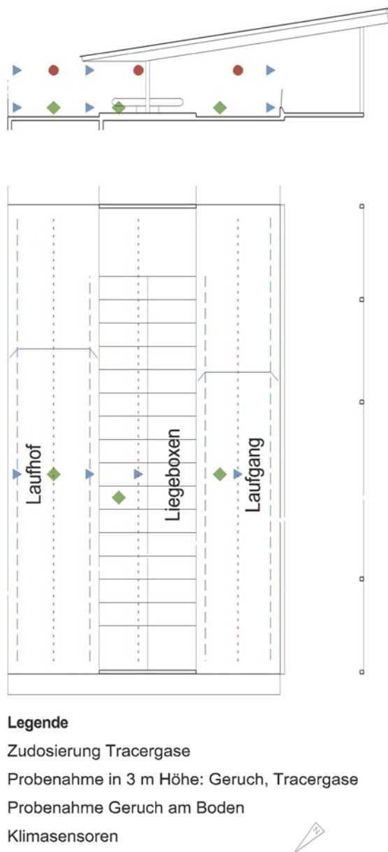
Abb. 2 | Schematische Darstellung mit Grundriss und Schnitt eines zweireihigen Liegeboxenlaufstalls mit Zudosierung, Probenahme sowie Klimasensoren.
