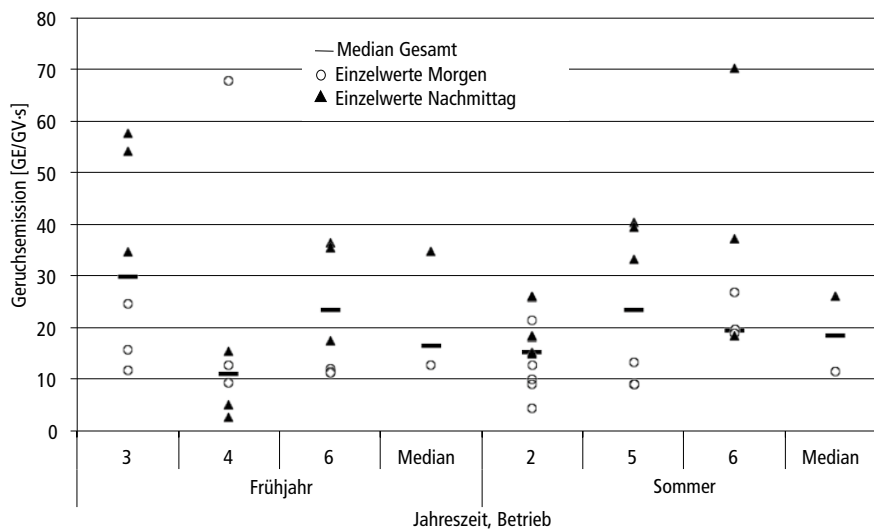
Abb. 5 | Geruchsemission, angegeben als Geruchseinheit pro Grossvieheinheit (entspricht 500 kg Lebendmasse) und Sekunde [GE/GV·s] als Einzelwerte am Morgen und Nachmittag, dargestellt pro Jahreszeit und Betrieb sowie als Median der Betriebe und pro Jahreszeit.
