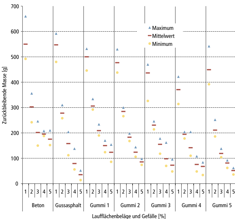
Abb. 4 | Zurückbleibende Masse bei unterschiedlichen Laufflächenbelägen und Gefällestufen.
