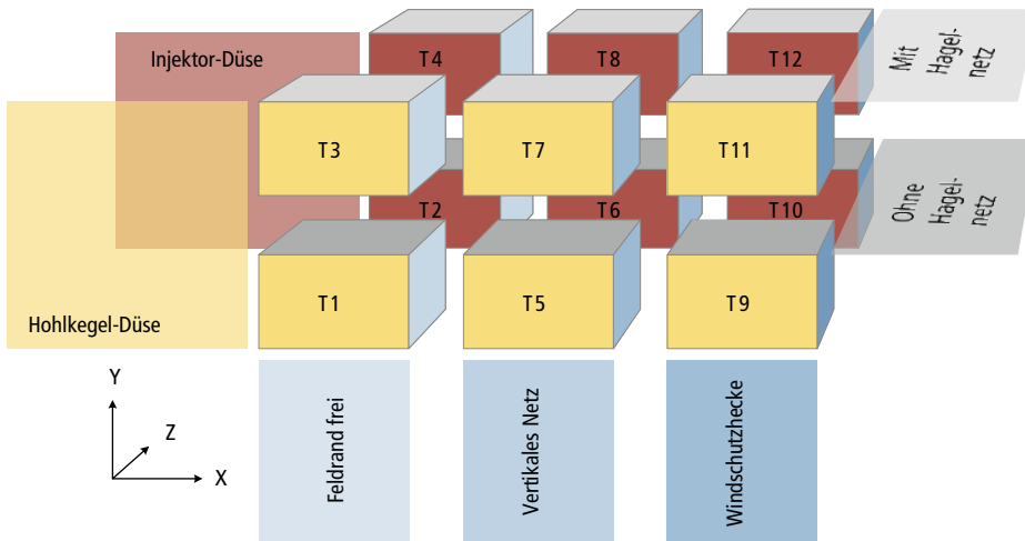
Abb. 4 | Darstellung aller Verfahren als dreidimensionale Matrix. Jede Box steht für ein Verfahren (T: Treatment), jede Ebene steht für eine Faktorstufe. X: Physische Barriere am Feldrand, Y: Physische Barriere über dem Feld, Z: Düsentechologie.
