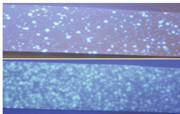
Abb. 3b | Kollektoren unter UV-Licht. Oben: Injektordüse. Unten: Hohlkegeldüse. Beide in 5 m Abstand vom Feldrand. (Foto: Stefan Wolf, Syngenta)
