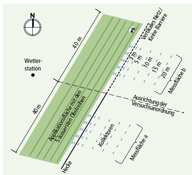
Abb. 2 | Versuchsaufbau, massstäbliche Darstellung.
