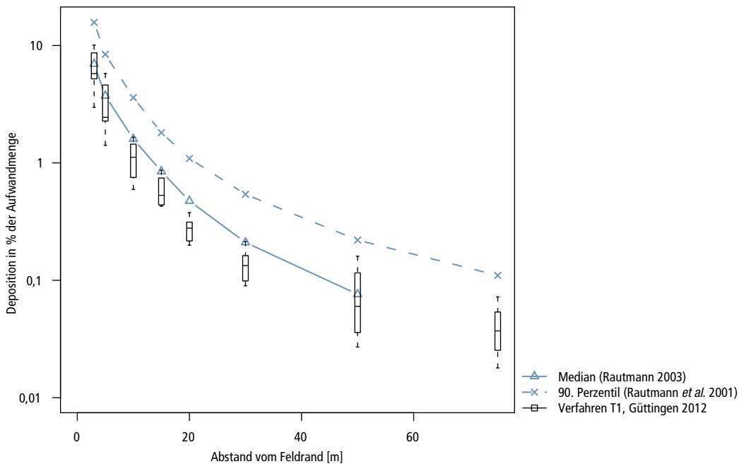
Abb. 6 | Vergleich der Depositionswerte in Göttingen (Verfahren T1) mit den Depositionsfunktionen (90. Perzentile und Mediane) nach Rautmann (Rautmann et al. 2001; Rautmann 2003).
